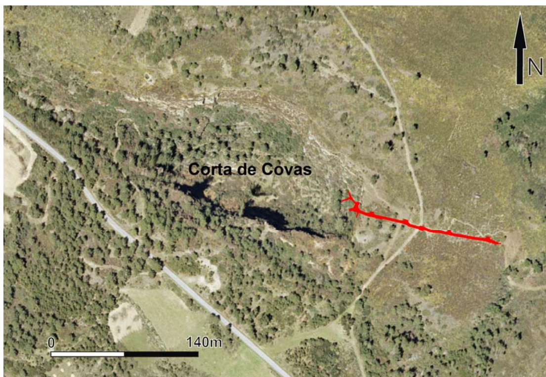
Abb. 5 Três Minas. Corta de Covas. Rot: Der unterirdische Verlauf der Galeria dos Alargamentos. Der Treppenschacht weicht von der Galerie nach Süden ab. (Ortofotomapa 1:5000 Câmara Municipal Vila Pouca de Aguiar. 3D-Laserscanaufnahme und Bearbeitung Helfert)
